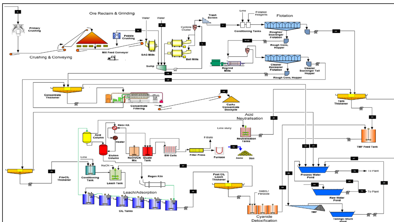
Слика 3: Дијаграм на тек на компонентите на проектот за бакар и злато „Иловица“
